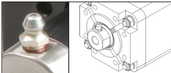
图 7.1：可以用适配的黄油嘴枪对 ServoWeld 电动缸进行重新润滑。执行这项操作，无需将电动缸拆下。
